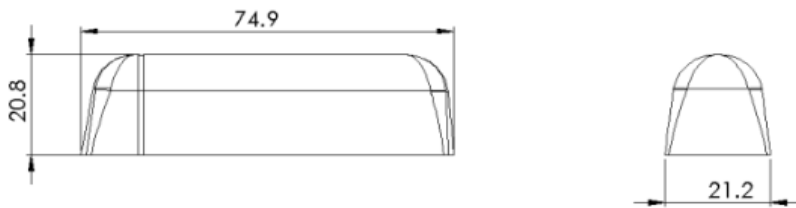
Dimensiones del sensor en mm
